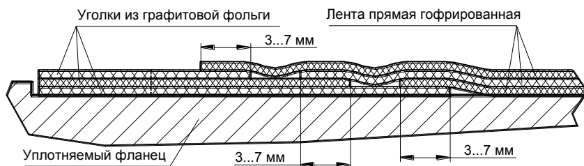
Рисунок Б.5.2 - Прокладка прямоугольная (вариант). После приклеивания уголков из графитовой фольги (см.рис.Б.5.1), приклеивается лента с нахлёстом 3...7 мм. На рисунке проказана прокладка из трех слоев.
