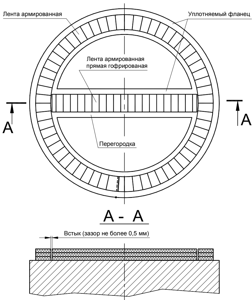
Рисунок Б.2 - Прокладка кольцевая с перегородкой.
